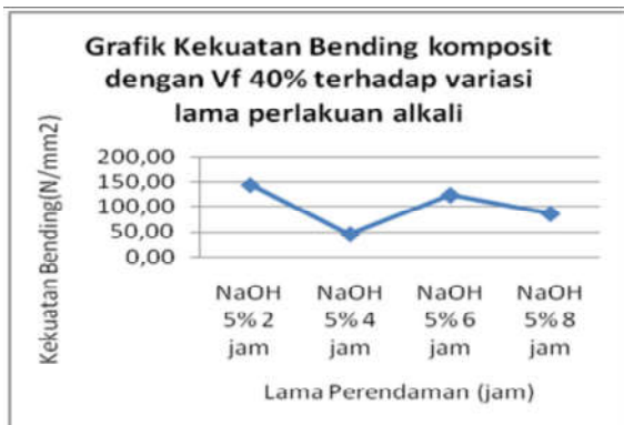
Gambar 2. Grafik kekuatan bending komposit dengan Vf = 40% terhadap variasi lama perlakuan alkali.
