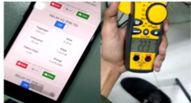
Gambar 5: Pengujian arus
