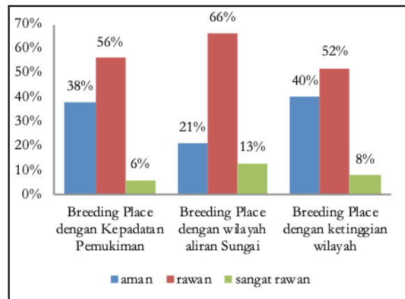
Gambar 19 Grafik parameter yang berpengaruh terhadap perkembangan Breeding Place di wilayah Kabupaten Bantul
