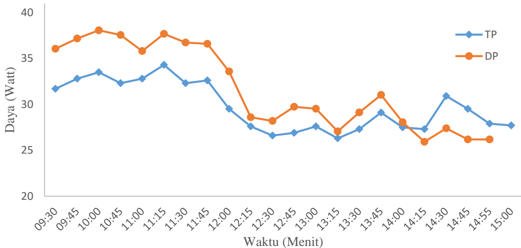
Gambar 7. Daya keluaran panel
