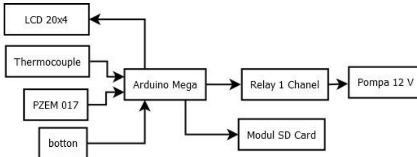
Gambar 4. Skema pengambilan datalogger
