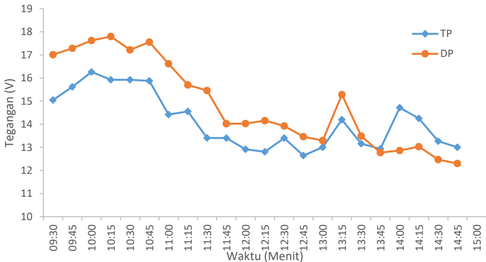
Gambar 6. Tegangan keluaran panel surya
