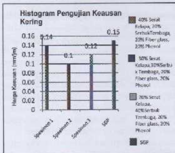
Gambar 1. Histogram Hasil Pengujian Keausan kering
