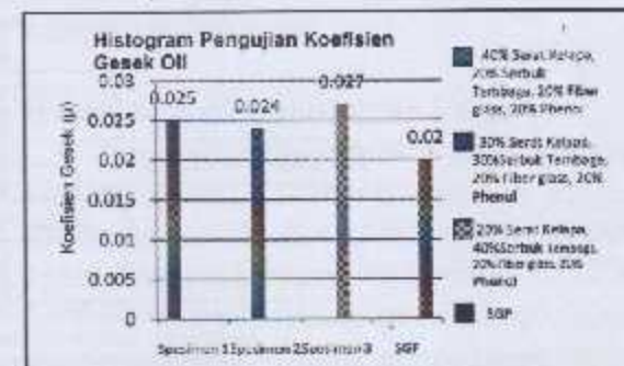
Gambar 4. Histogram Hasil koefisien gesek oli
