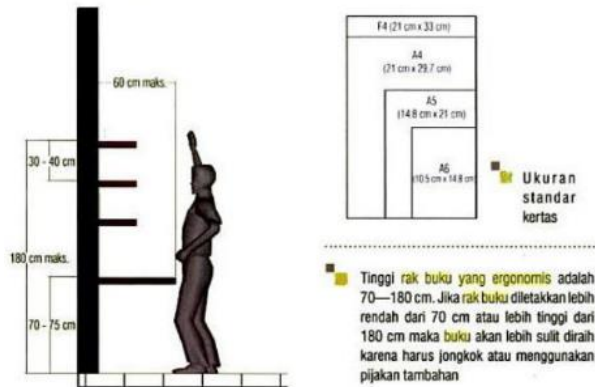
Gambar 4. Standar ukuran rak buku ideal (Sumber : Swasty, 2010)
