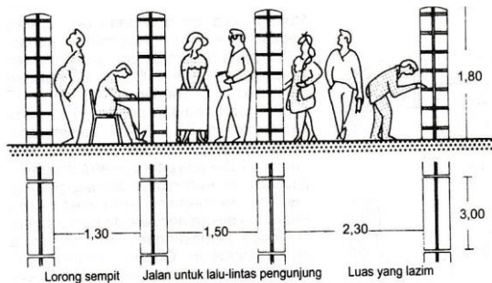
Gambar 5. Jarak sirkulasi rak buku (Sumber : Neufert, 2002)
