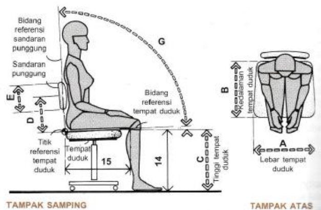
Gambar 8. Kursi kerja yang ergonomis (Sumber : Panero, 1979)
