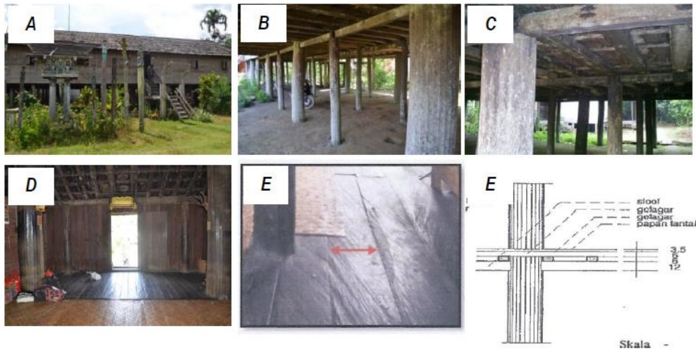
Gambar 2. (a) tampak depan betang toyoi, (b) konstruksi tiang pada bangunan betang toyoi, (c) konstruksi tiang, tongket, bawat, dan gegahan, (d) bentuk lantai pada bangunan betang toyoi, (e) detail elemen lantai pada betang toyoi (Sumber : Usop, 2014)
